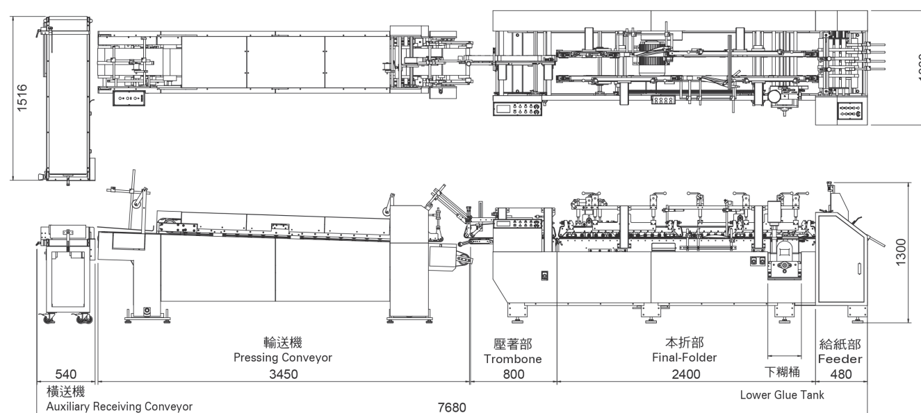
外型基礎圖 Floor Plan
